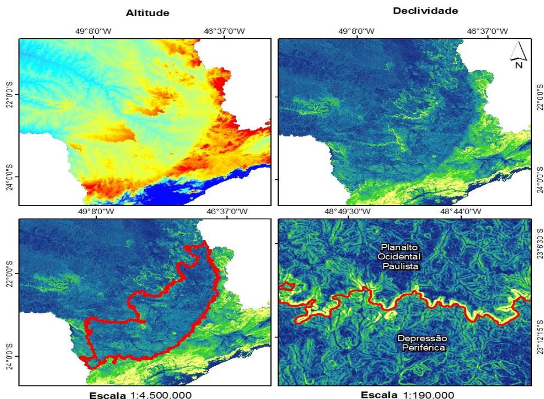
Figura 2. Dados utilizados para a delimitação da divisa entre a Depressão Periférica e o Planalto Ocidental Paulista.
