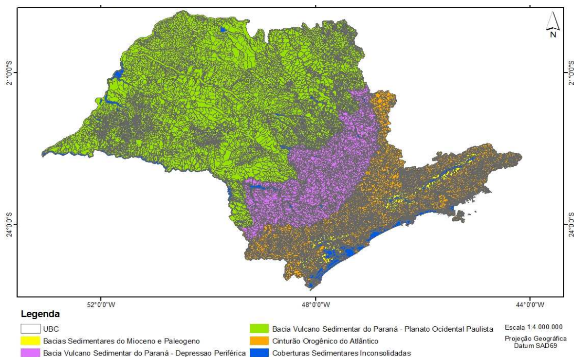
Figura 20 - UBC para o Estado de São Paulo agrupadas em cinco categorias morfoestruturais.
