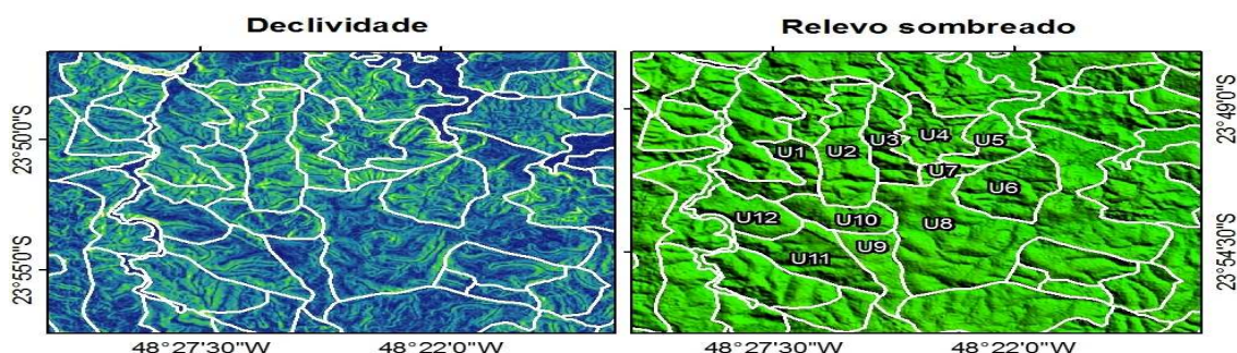
Figura 5. Área da Depressão do Paranapanema compartimentada em UBC.
