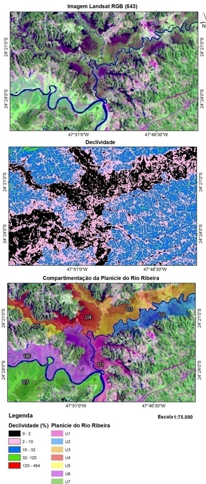
Figura 14. Exemplo de compartimentação da planície do rio Ribeira.
