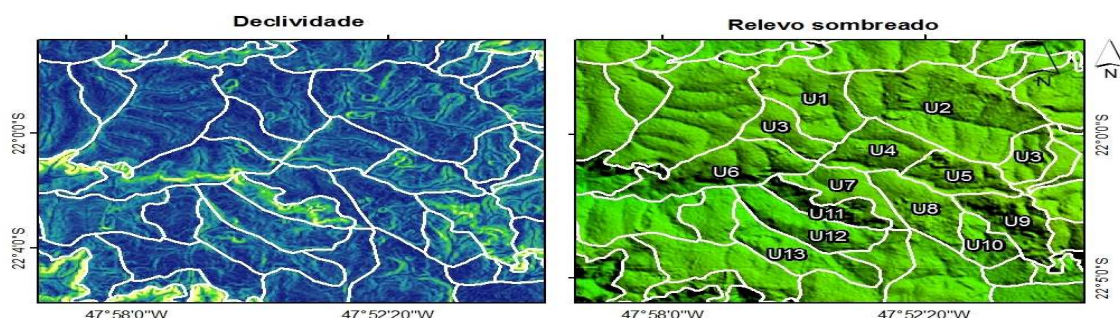
Figura 7. Área compartimentada em UBC no Planalto Residual de São Carlos.
