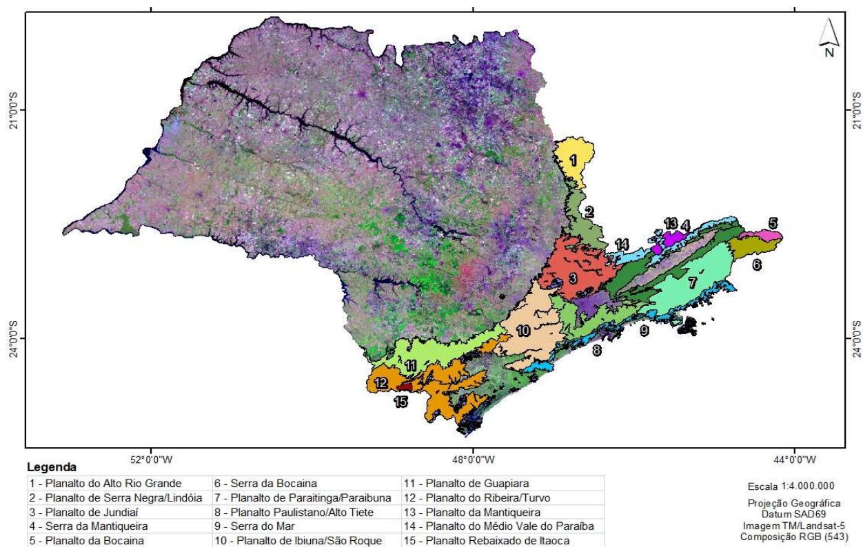
Figura 25 – Detalhamento dos níveis hierárquicos do Planalto Atlântico.
