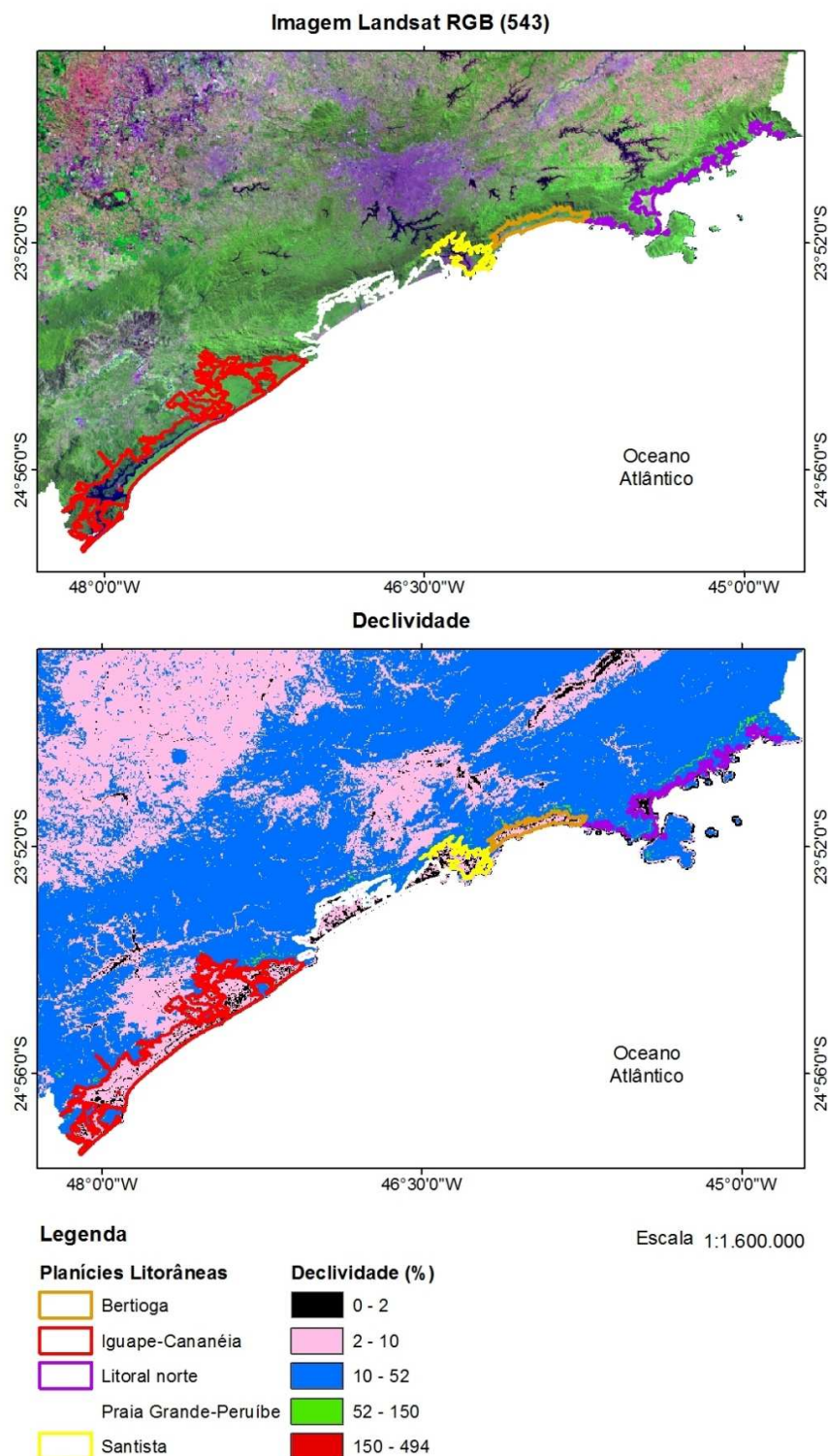
Figura 15. Distribuição das planícies litorâneas do Estado.
