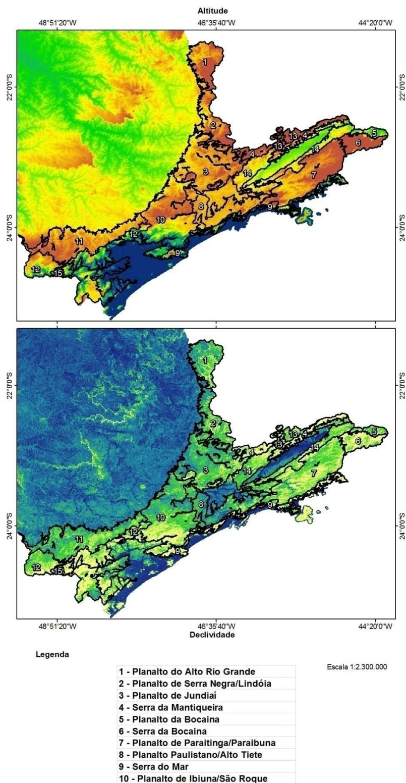
Figura 18. Principais compartimentos localizados no Cinturão Orogênico.
