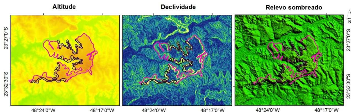
Figura 4. Morro isolado localizado na depressão indiferenciada.
