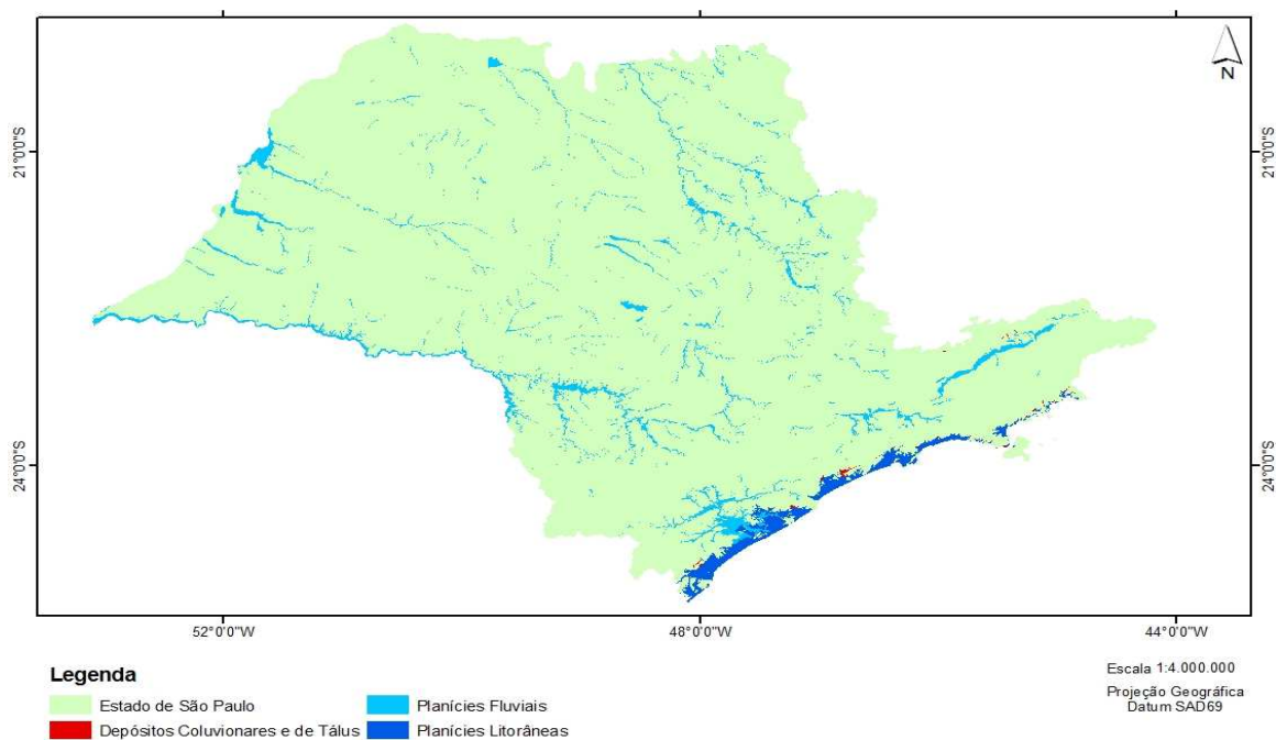
Figura 21 - Detalhamento dos níveis hierárquicos das Coberturas Sedimentares Inconsolidadas.
