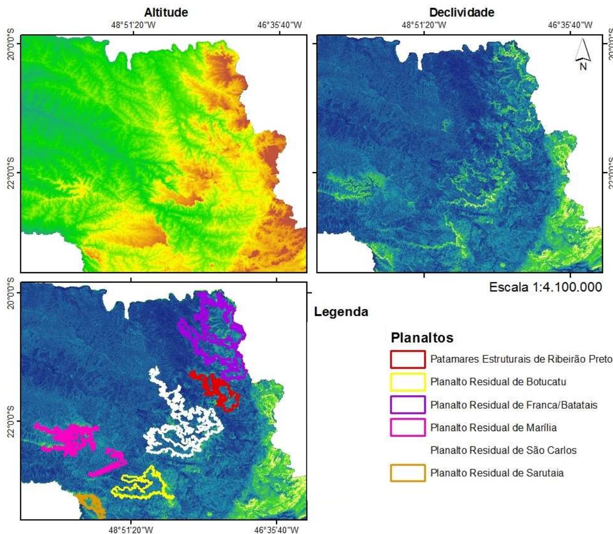
Figura 6. Planaltos localizados no Planalto Ocidental Paulista.
