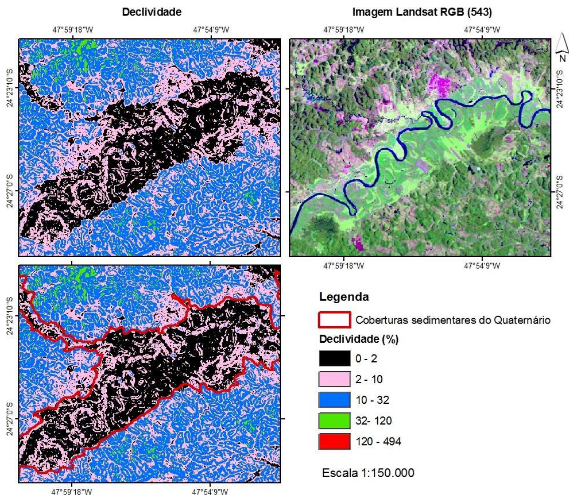
Figura 11. Principais dados utilizados para identificação e vetorização das planícies das coberturas sedimentares inconsolidadas do Quaternário.
