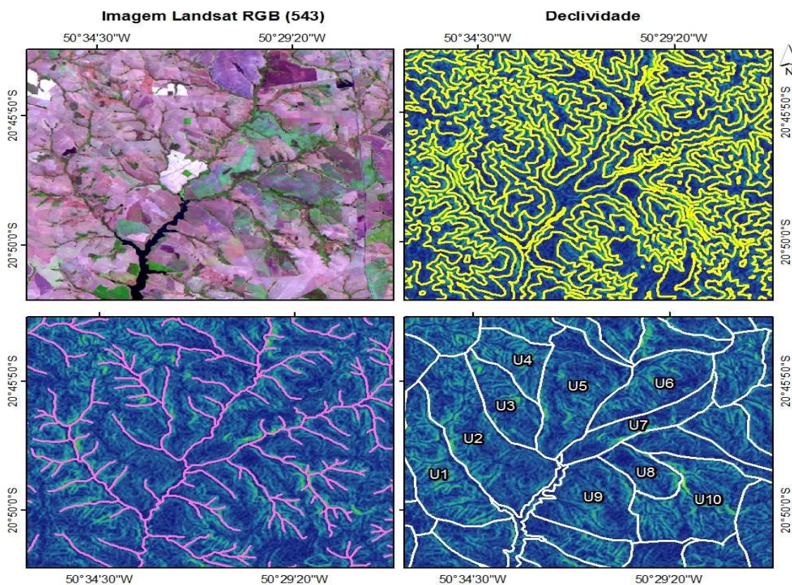
Figura 8. Área compartimentada em UBC no Planalto Ocidental Paulista.
