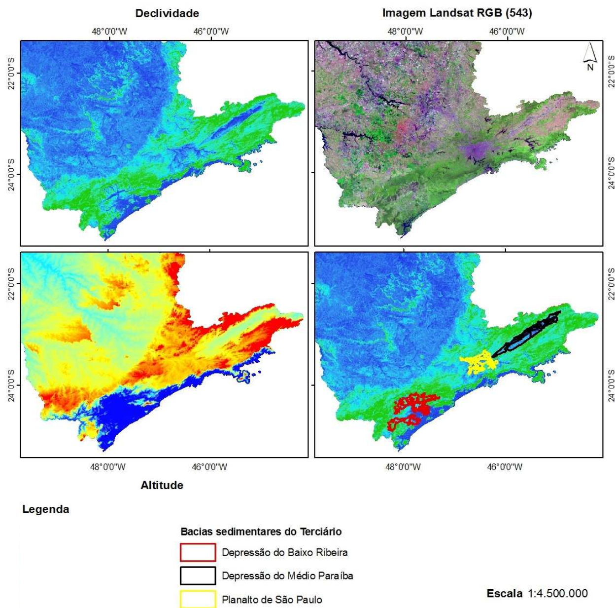
Figura 9. Representação dos principais dados utilizados para a vetorização das bacias sedimentares do Mioceno e Paleógeno (Terciário).
