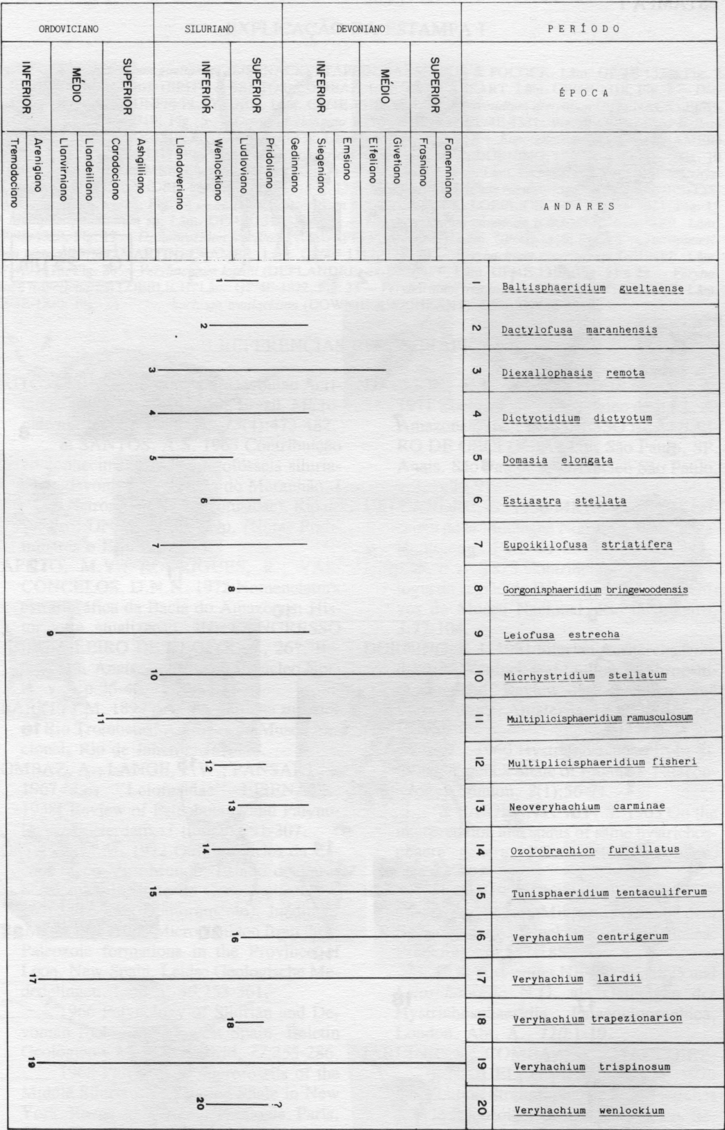
FIGURA 2 — Distribuição cronológica das espécies identificadas (baseada em LISTER, 1970; LOEBLICH, 1970; THUSU, 1973; JARDINÉ et al. , 1974 e DORNING, 1981).
