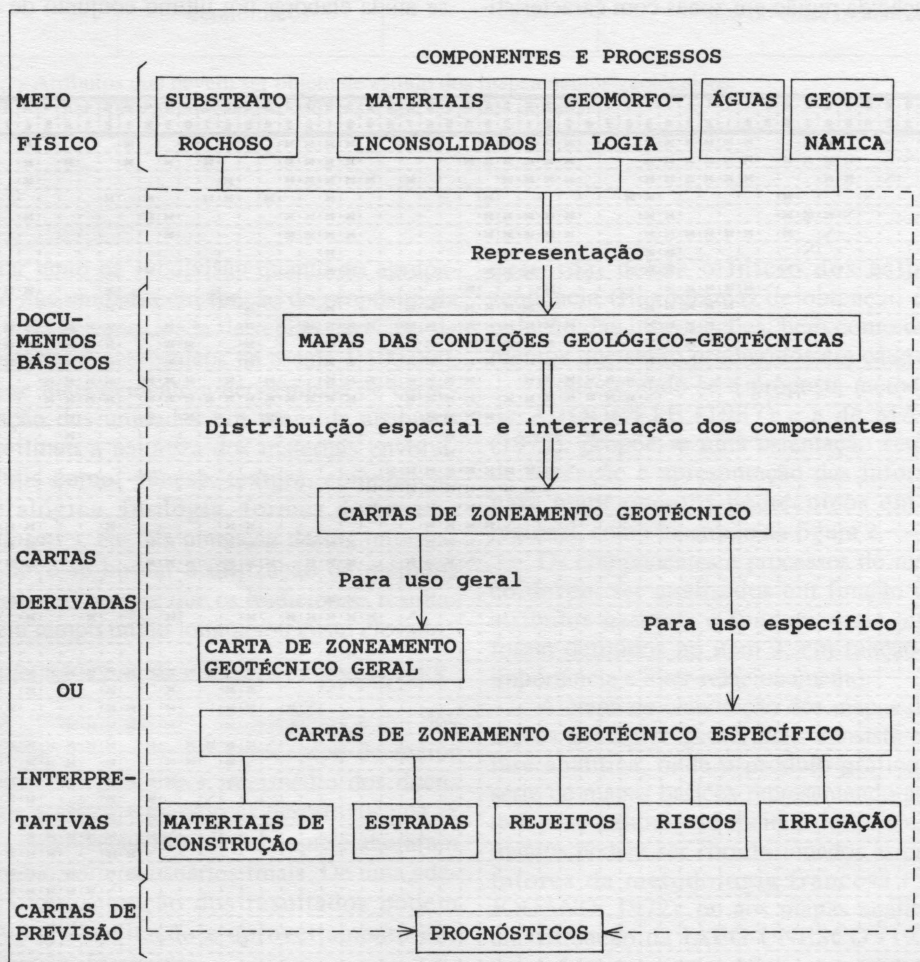
Figura 2 – Fluxograma de obtenção e apresentação das informações do meio físico em mapeamentos geotécnicos regionais (adaptado de MATULA, 1979).
