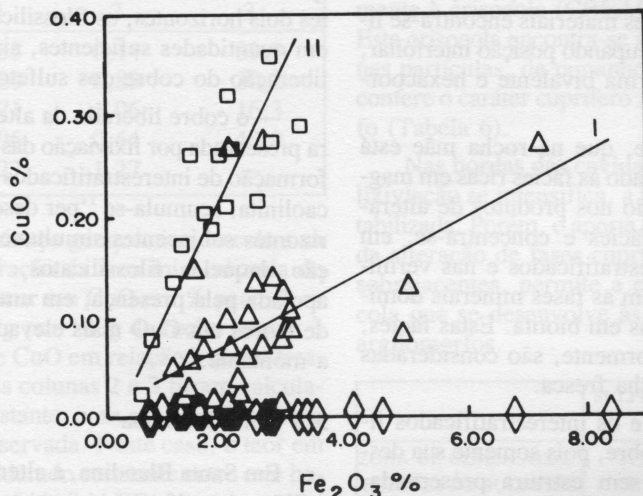
FIGURA 5 — Correlação \text{Fe}_2\text{O}_3 — \text{CuO} no horizonte rocha alterada coerente (RAC) do perfil de Chapada Grande. IA ( R = 0,53 ); II Ó ( R = 0,82 ).
