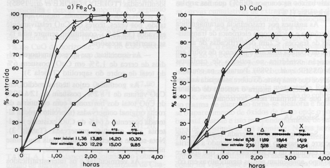
FIGURA 6 — Curvas cumulativas do Fe_2O_3 e do CuO, extraídos pelo reativo oxálico, sob radiação ultravioleta, para os materiais de Chapada Grande. 100% = total de elementos na fração < 2\mu m .
