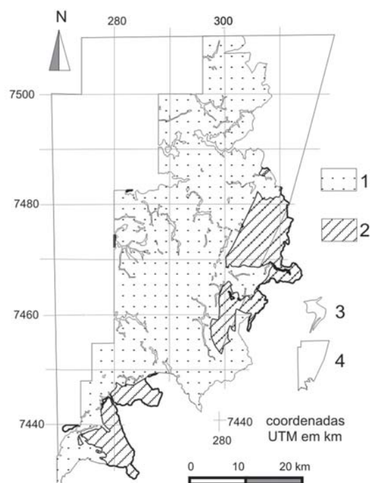
FIGURA 6 - Domínios onde a cobertura de superfícies aplainadas (TQsp) tende a ocorrer ou estar ausente (modificado de INSTITUTO GEOLÓGICO 2002). (1) Domínio onde a cobertura TQsp tende a ocorrer, (2) Domínio onde a cobertura TQsp tende a estar ausente, (3) Planície aluvial, (4) Limite da área de estudo.
